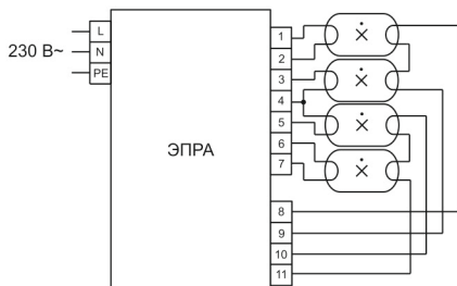
Рисунок 4. Электрическая схема подключения ЭПРА 418
