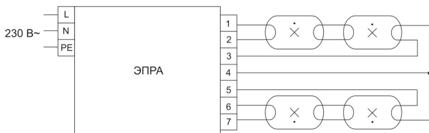
Рисунок 5. Электрическая схема подключения ЭПРА 418М
